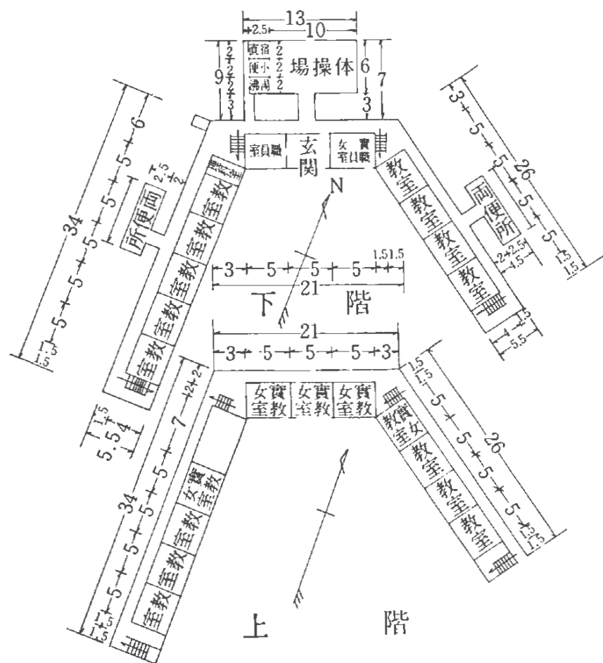
第13図 七戸尋常高等小学校第二校舎平面図（大正14年）
