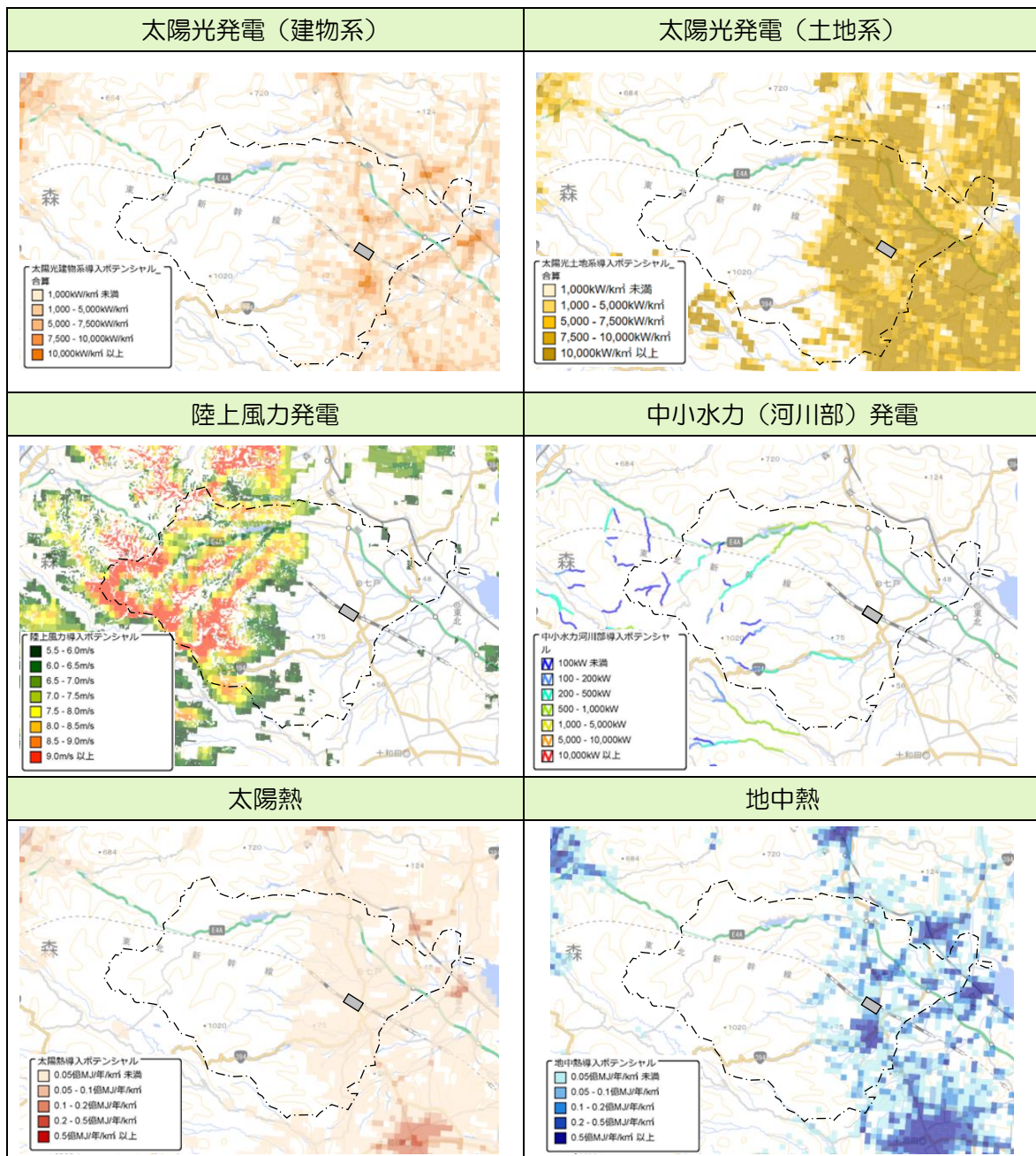
図@@ 各種再生可能エネルギー導入ポテンシャルマップ
