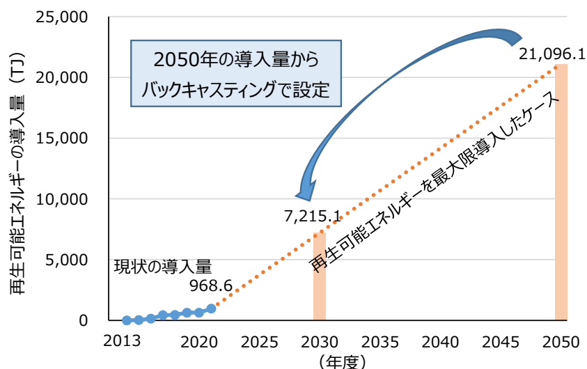
図@@ 再生可能エネルギー導入量（最大限導入ケース）の推移
