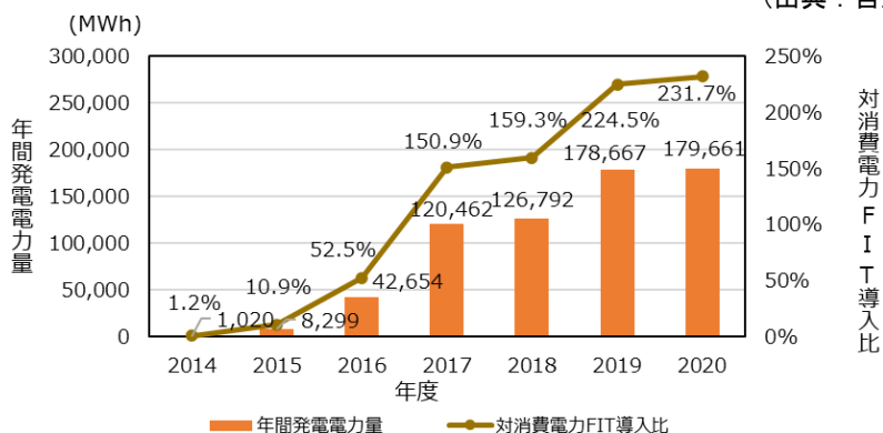
図@@ 再生可能エネルギーの年間発電電力量の経年変化
