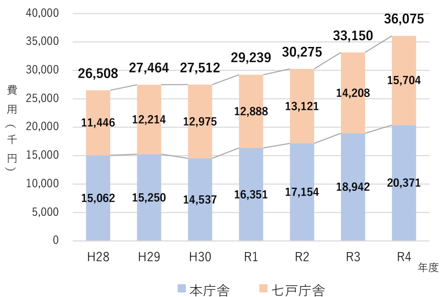
【七戸町役場本庁舎及び七戸庁舎 年間維持管理費の推移】
