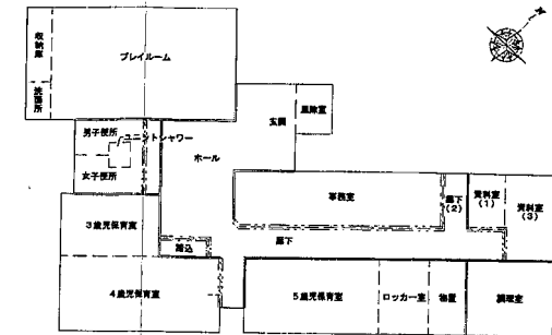
改修後間仕切壁キープラン S=1/200
