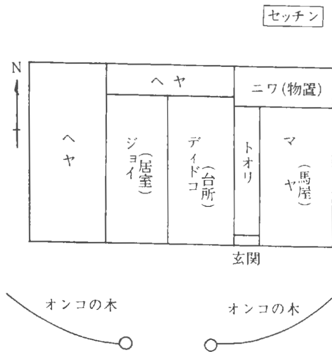
第3図 一般農家の住居構造例
