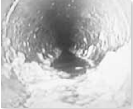
天間林地区内の管渠内部
